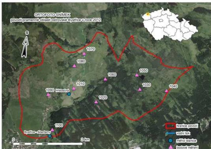
Obr. 2: Schematická mapa povodí s vyznačenými měřicími stanicemi a s polohou systematicky měřených bodů
