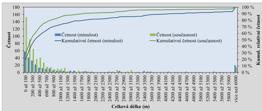
Obr. 3: Histogram četností délek skupin úseků toků nepřerušených vodní nádrží pro obě uvažovaná časová období.
