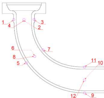
Obr 7: Schéma rozmístění tlakových sond
