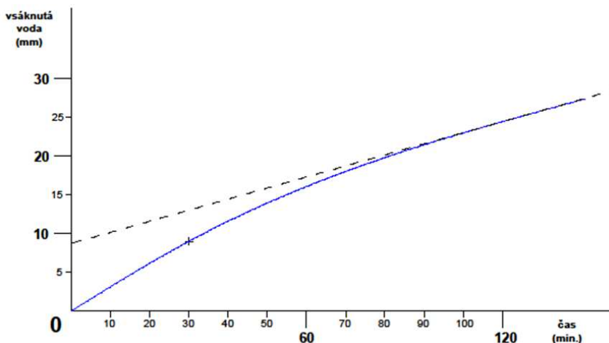
Graf 3: sonda č. 3 (čárkovaně rychlost vsakování v čase 120 minut = 8,55 mm/h)
