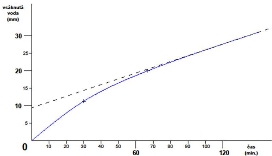
Graf. 2.: sonda č. 2 (čárkovně rychlost vsakování v čase 120 minut = 9,9 mm/h)
